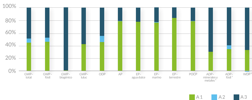
Distribución de cada parámetro DAP entre las distintas etapas del proceso de producción de áridos naturales. Fuente: DAP FdA.
